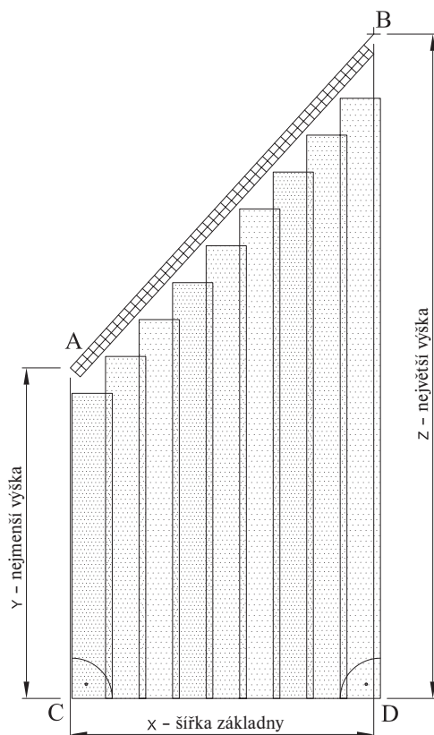
Vertikální žaluzie Blue Line – vyměření šikmého provedení
